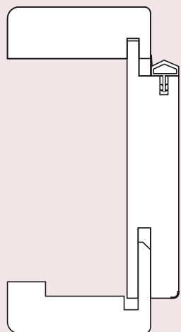
Durchgang mit schlagfester ABS-Starkkante
